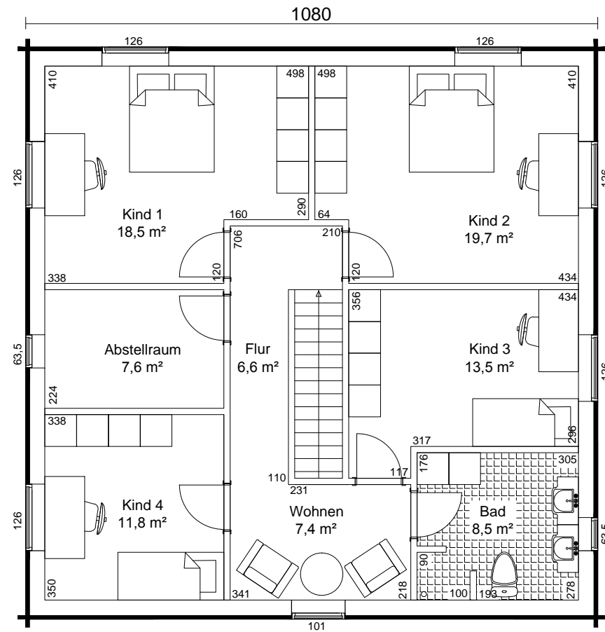
Obergeschoß 117 m 2
