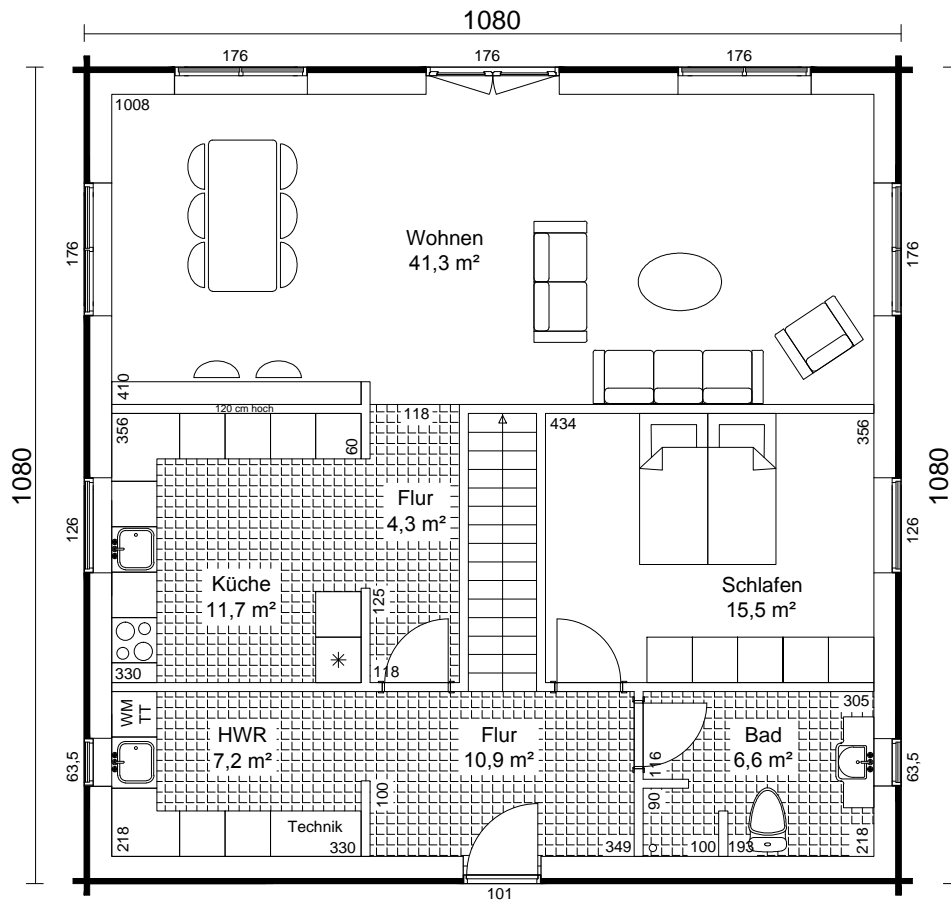
Erdgeschoß 117 m 2
